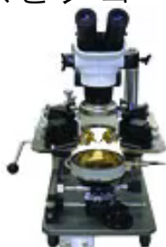
▲小型マニュアルプローバー
