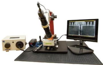
▲卓上型マニュアル劈開装置
