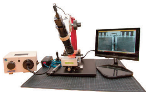
▲卓上型マニュアル劈開装置
