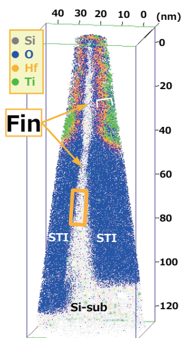
NMOSの3DAP像
