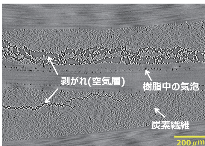
3次元X線顕微鏡像(任意断面)
